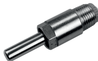
10092-14 a 200 Humedecedora 1/2" para cerdas, caudal agua max 12 ltr/ min., con rosca macho 1/2"
